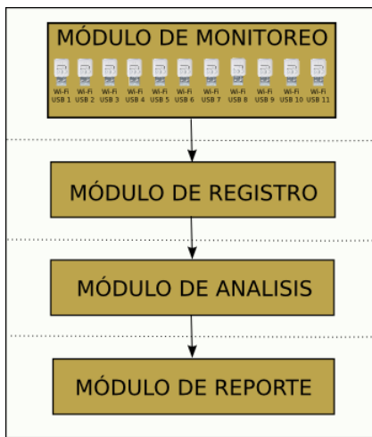
Figura 2: Diagrama de bloques de la arquitectura de sniffer propuesto.
