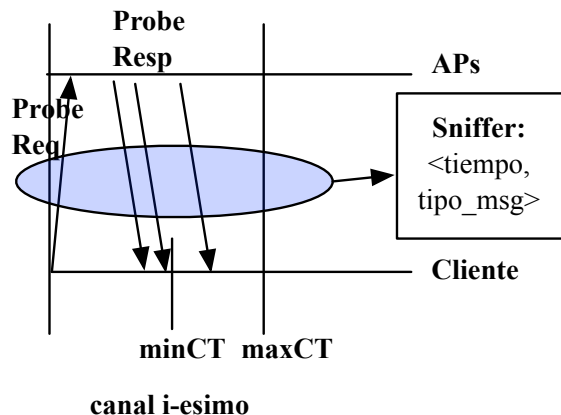
Figura 1: Bosquejo de red IEEE 802.11 con un sniffer.
