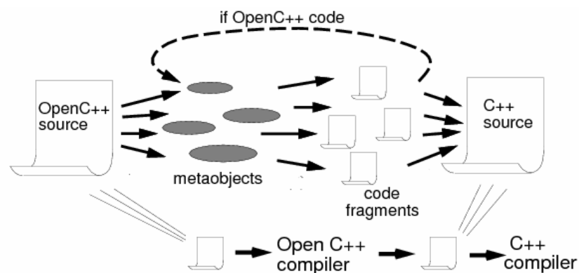
Figura 10. Esquema de manejo de Open C++ (tomado de [36])
