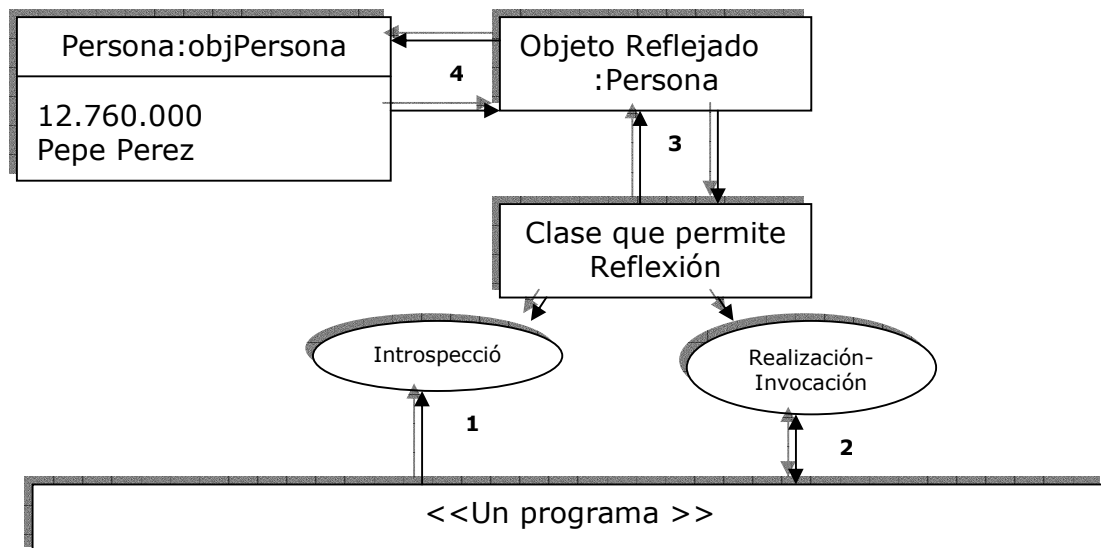
Figura 11. Un ejemplo de Solución Reflexiva en C++
