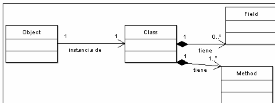
Figura 31. Modelo Conceptual de SIRC
